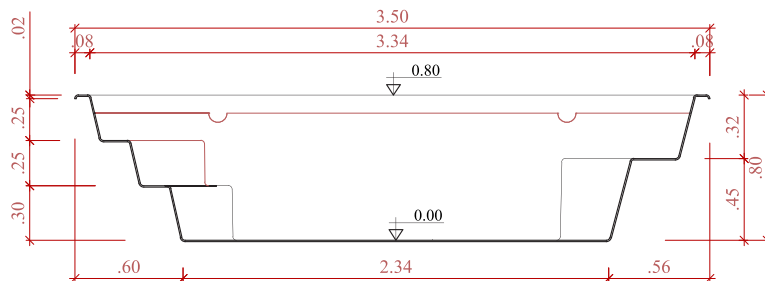
CORTE LONGITUDINAL
