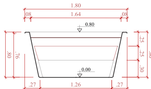
CORTE TRANSVERSAL ESCALA 1:30
