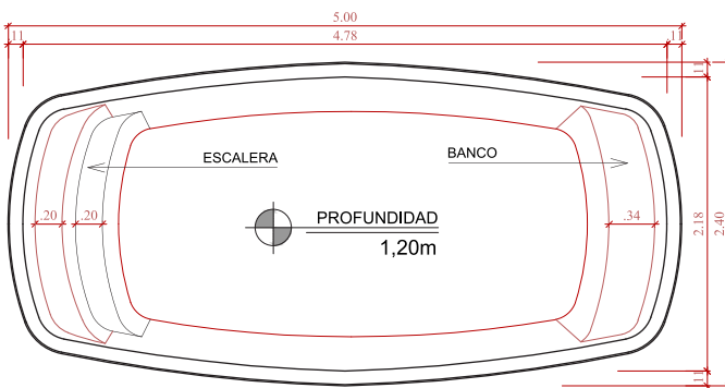
DIBUJO TÉCNICO ESCALA 1:50
