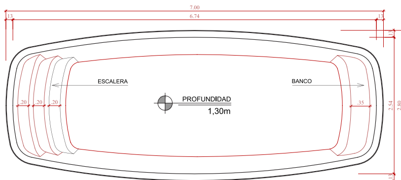
DIBUJO TÉCNICO ESCALA 1:50
