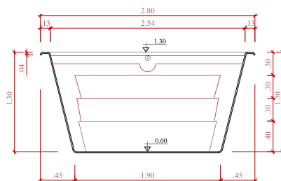
CORTE TRANSVERSAL ESCALA 1:50
