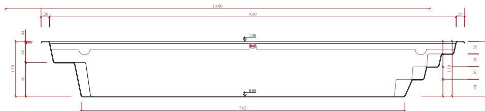
CORTE LONGITUDINAL ESCALA 1:50
