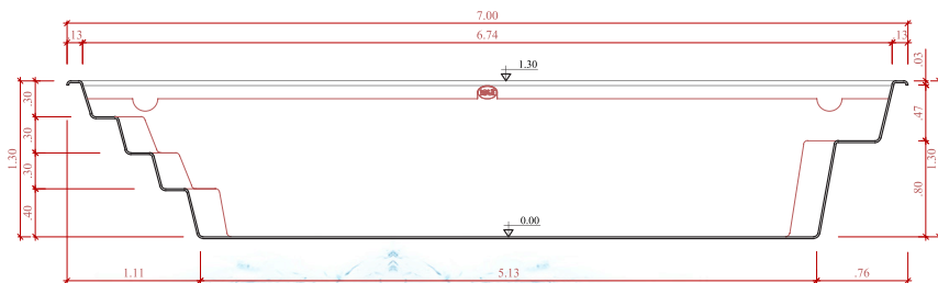
CORTE LONGITUDINAL ESCALA 1:50
