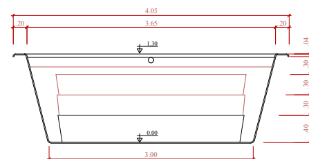
CORTE TRANSVERSAL ESCALA 1:50
