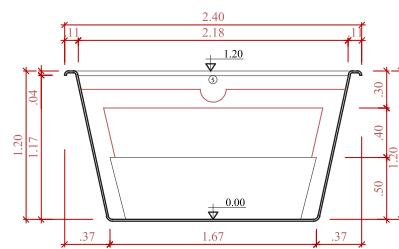
CORTE TRANSVERSAL ESCALA 1:50
